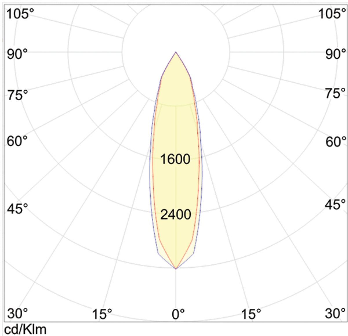
5270 - 14° Lens (.9N)
