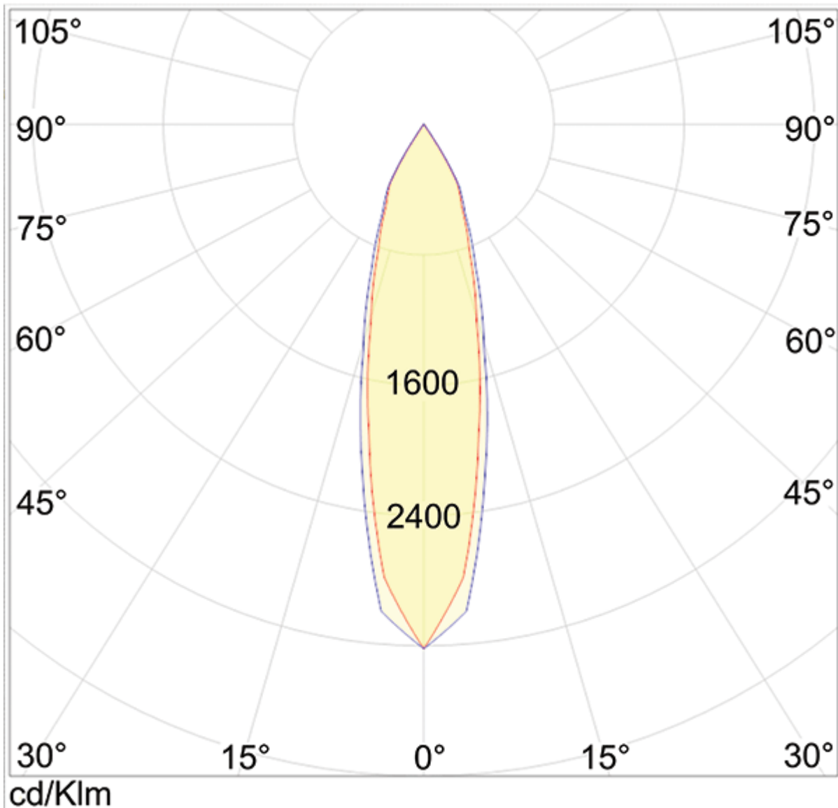
5270 - 14° Lens (.9N)
