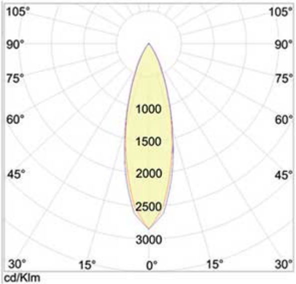
5243 - 13° Lens (.9N)
