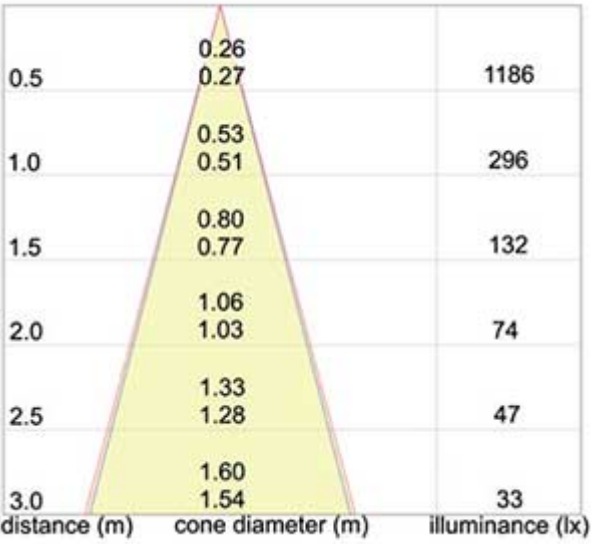
5243 - 31° Lens (.9)
